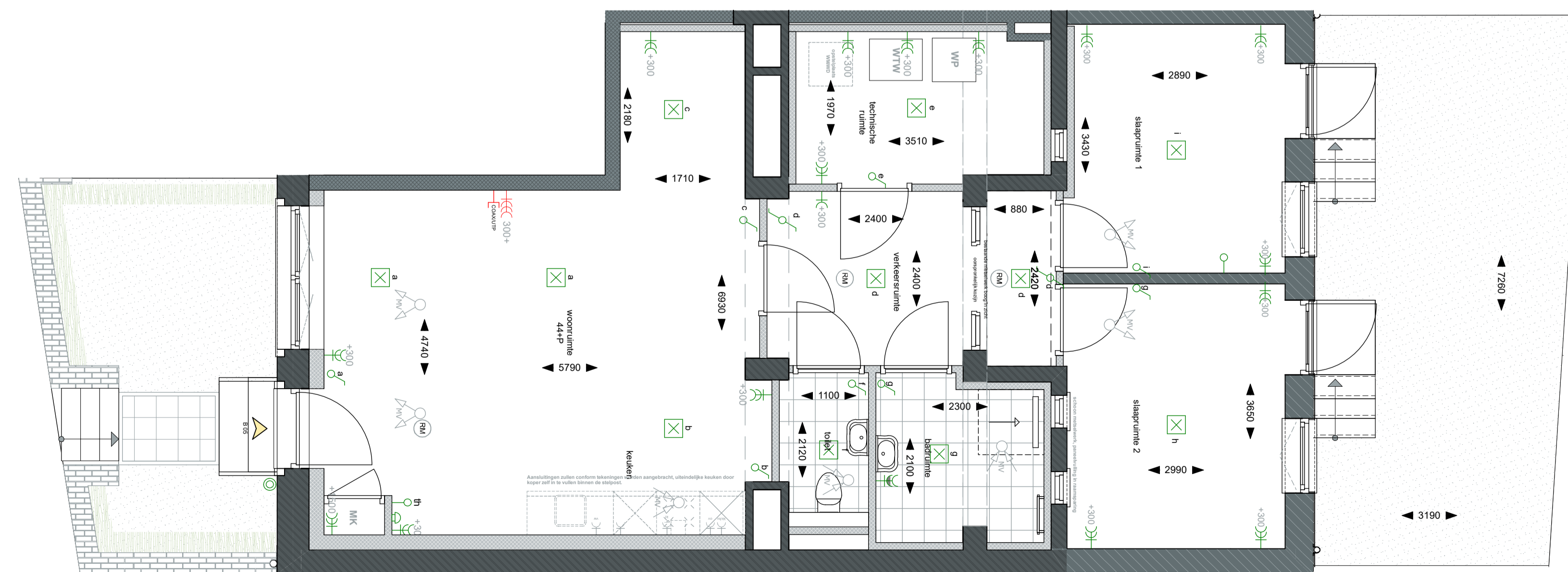
Begane grond - 1:50
